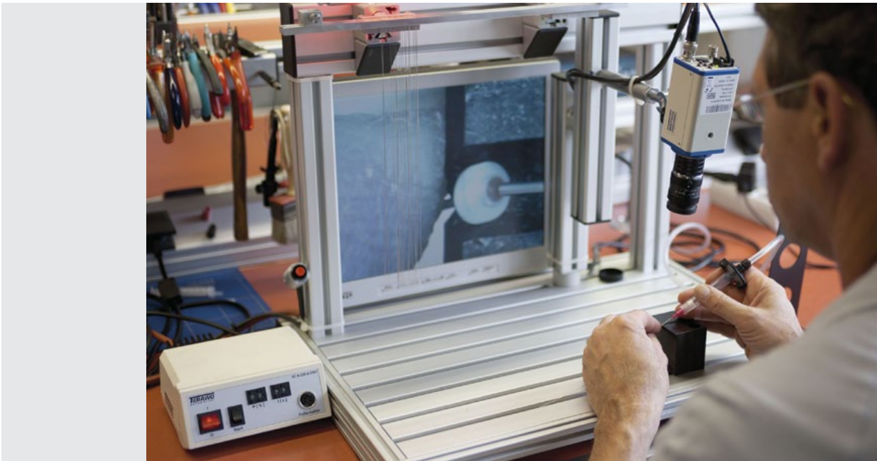
Arbeitsplatz mit Kamera aus item Profilen des MB Systembaukastens.
